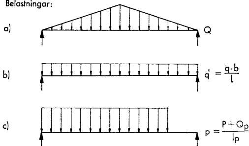
Fig. 16:3. Belastningsdiagram för beräkning av bärande konstruktioner över dörr- och fönsteröppningar.
