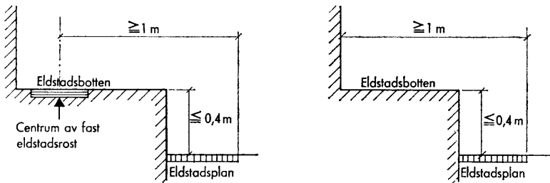
Fig. 35:1. Eldstadsplan framför öppen spis.
