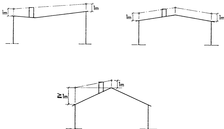
Fig. 35:2. Rökkanals höjd över tak.
