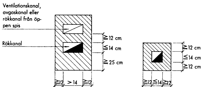
Fig. 35:4. Väggtjocklek hos skorstenar av tegel.
