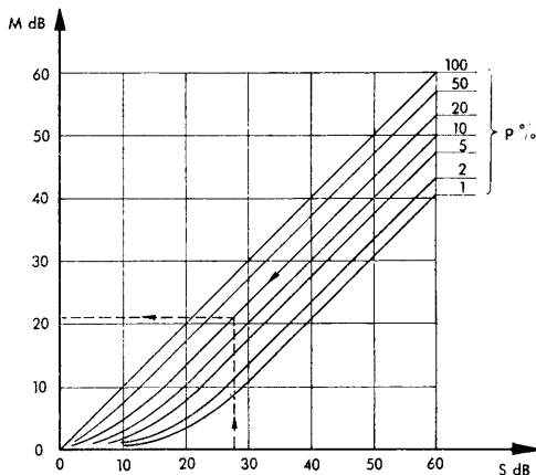
Fig. 23:3. Nomogram för beräkning av resulterande isolering.
