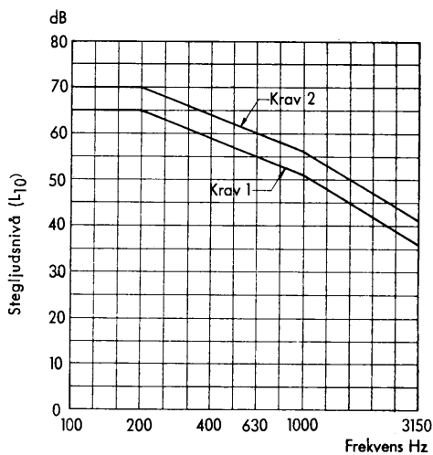
Fig. 23.2. Maximikurvor för stegljudsnivån enligt tabell 23.2.
