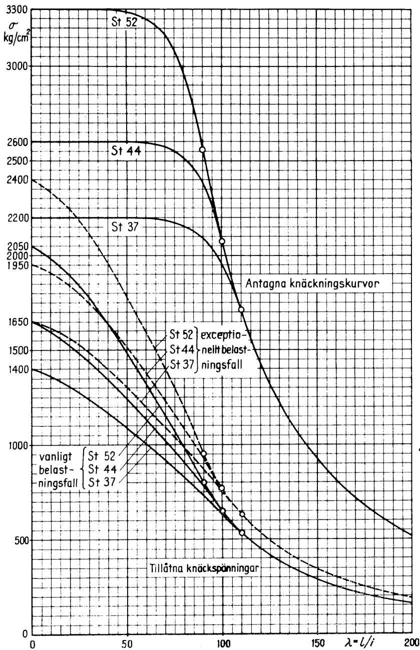
Fig. 14.2. Tillåten påkänning vid knäckning (tillåten knäckspänning) för St 37, St 44 resp. St 52 då \sigma_{till} vid vanligt belastningsfall är 1400, 1650 resp. 2050 kg/cm 2 .
