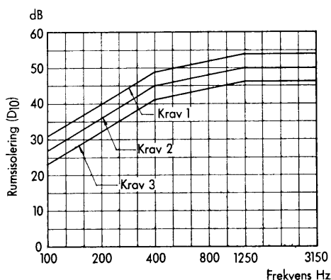
Fig. 23:1. Minimikurvor för rumsisoleringen mot luftljud enligt tabell 23:1.
