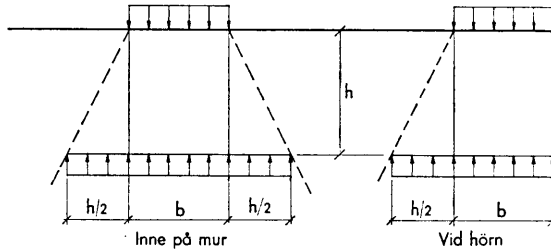
Fig. 16:2. Tryckutbredning under upplag.
