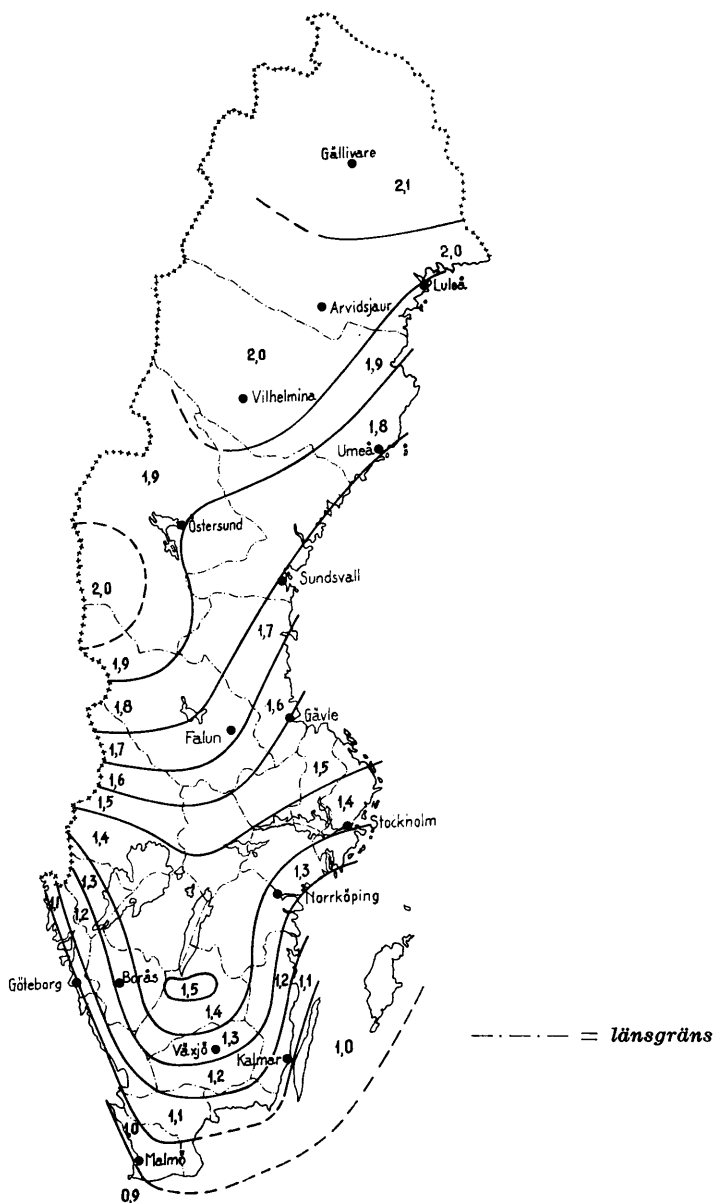
Fig. 13:1. Frostfri nivå för byggnadsgrunder. Siffrorna anger ungefärligt djup i meter till frostfri nivå.
