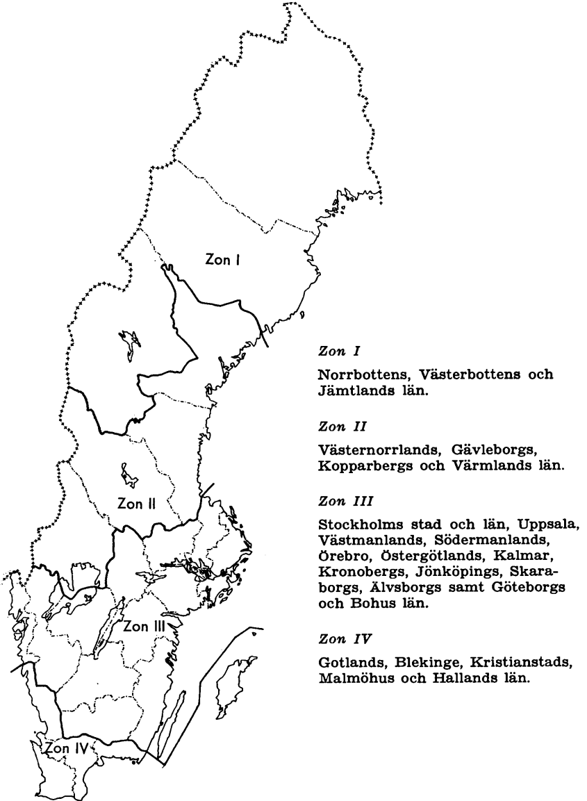
Fig. 22:1. Zonindelning med hänsyn till kraven på värmeisolering (jfr tabell 22:1).
