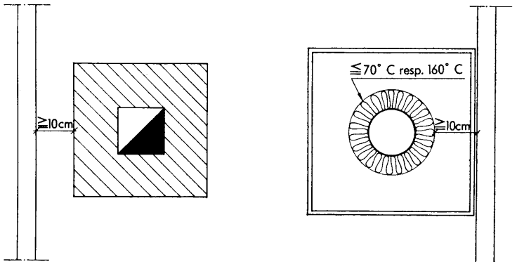
Fig. 35:3. Avstånd mellan rökkanal och brännbart material.
