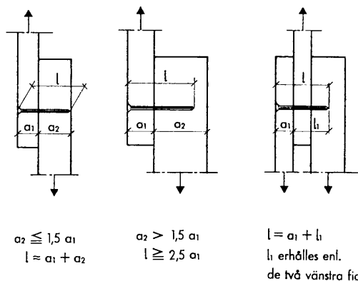
Fig. 17:5. Erforderlig spiklängd vid olika förband.
