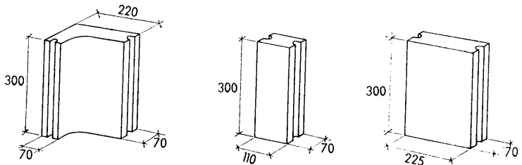
Fig. 35:5. Höganäs fodertegel. Mått i mm.
