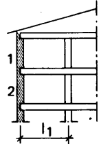
Figur 24:422 b – c Faktor vid väggar med från en sida anslutande bjälklag (ytterväggar och liknande). Nomogram b gäller vid korsarmerade bjälklag med minsta spännvidden max 5,0 m. Nomogram c gäller vid enkelspända bjälklag \leq 5,0 m.
