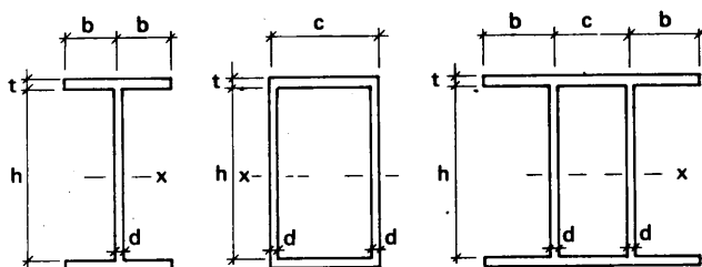
Figur 28:21 Beteckningar för tvärsnittsmått.
