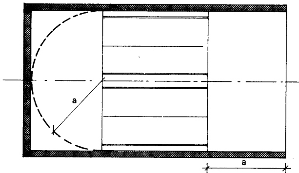
Figur 62:23 Trappplans bredd
