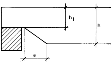
Figur 27:332 Inskäring vid upplag.
