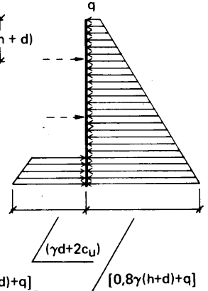
Figur 21:422 a – b Jordtrycksfördelning vid spontvägg med a) en förankrings- eller avsträvningsnivå samt b) flera förankrings- eller avsträvningsnivåer.
