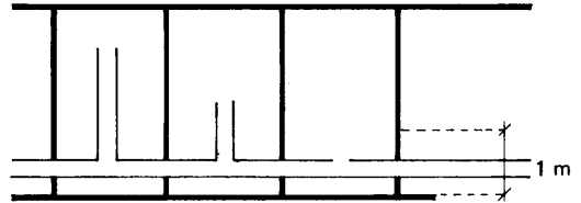
Figur 52:341 b Anslutning till samlingskanal som betjänar flera brandceller.
