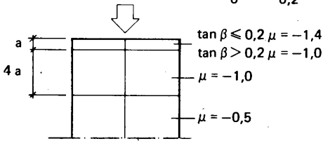
Figur 21:6332 a Formfaktorer för utvärdig vindlast på sadeltak och höjd h för bestämning av hastighetstryck enligt :62. Undertryck betecknas negativt, övertryck positivt.
