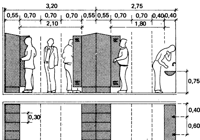
Figur 64:3 a Minsta godtagbara fria utrymmen vid klädskåp och tvättränna. Mått i meter.
