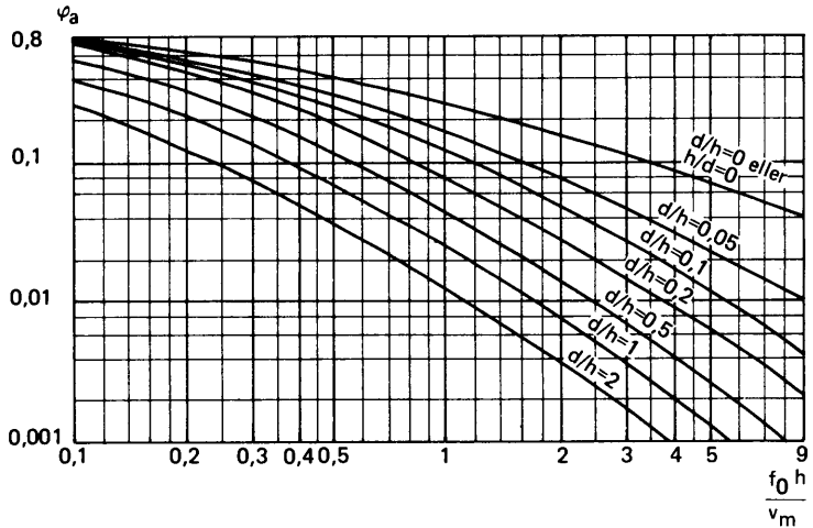
Figur 21:642 d Vindlastens storleksfaktor som funktion av f_0 h/v_m med egenfrekvensen för grundsvängningen f_0 , den anblåsta konstruktionens höjd h , dess största tvärrmått d och vindens medelhastighet v_m .
