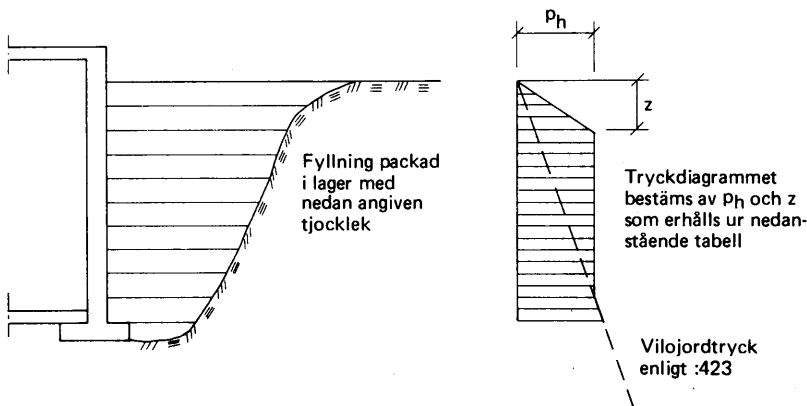
Figur 21:451 Jordtryck vid packad återfyllning av friktionsjord.
