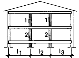
Figur 24:422 f–g Faktor vid väggar med från båda sidor anslutande bjälklag (innerväggar) eller då e/b är känt.
