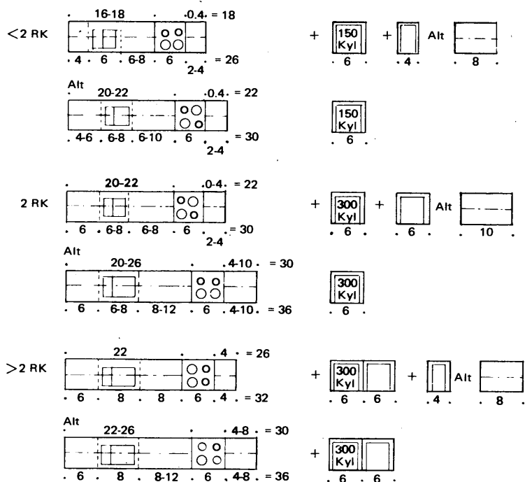
Figur 71:214 Köksutrustningsmängd för olika lägenhetsstorlekar. Delmått anges i dm.
