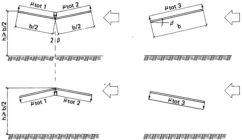
Figur 21:634 Formfaktor \mu_{tot} för skärmtak som lutar vinkeln \beta mot horisontalplanet. \beta antas vara > 5^\circ .
