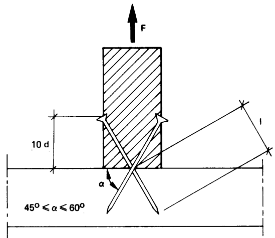
Figur 27:2223 b Skråspikning.
