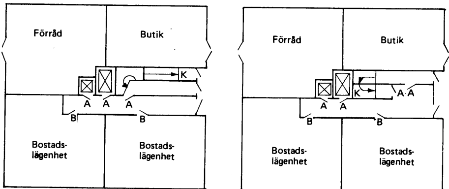
Figur 37:212 Principskisser med exempel på entréväning vid brandsäkert trapphus i bostadshus. A betecknar dörr i lägst klass A 60, B dörr i lägst klass B 30 och K betecknar källartappa.
