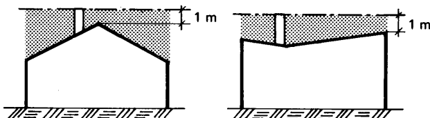
Figur 44:121 Rökkanals höjd över tak om ansluten eldstad har en tillförd värmeeffekt av högst 60 kW.
