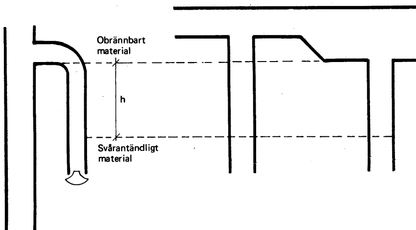
Figur 52:344 Princip för anordnande av röklås.
