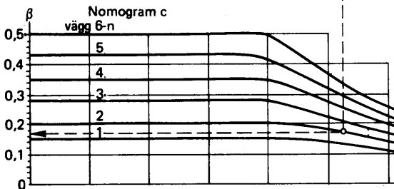
Figur 24:422 b – c Faktor vid väggar med från en sida anslutande bjälklag (ytterväggar och liknande). Nomogram b gäller vid korsarmerade bjälklag med minsta spännvidden max 5,0 m. Nomogram c gäller vid enkelspända bjälklag \leq 5,0 m.
