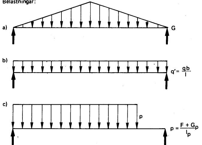
Figur 24:41 b Laster för beräkning av bärande konstruktion över öppning.
