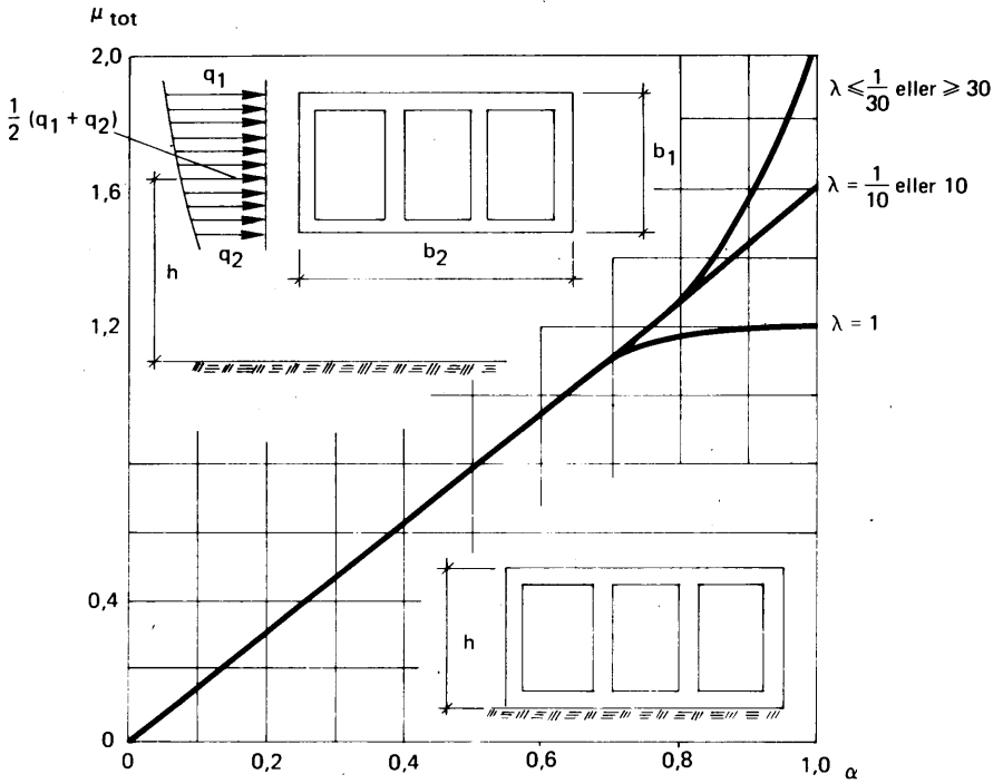
Figur 21:6342 a Formfaktor för en skärm med kantiga stänger. \alpha = A_p/A där A_p är nettoarean av anblåsta stänger i skärmen och A är skärmens bruttoarea. \lambda = b_1/b_2
