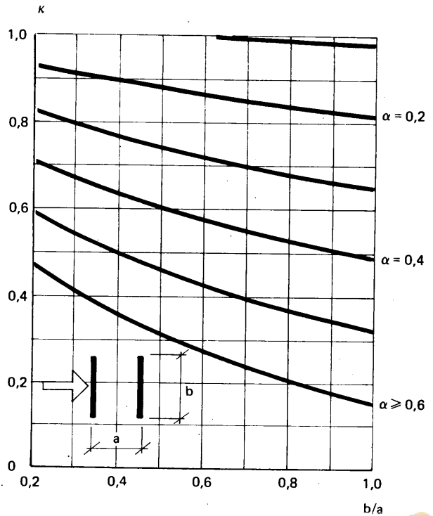
Figur 21:6342 a Formfaktor för en skärm med kantiga stänger. \alpha = A_p/A där A_p är nettoarean av anblåsta stänger i skärmen och A är skärmens bruttoarea. \lambda = b_1/b_2
