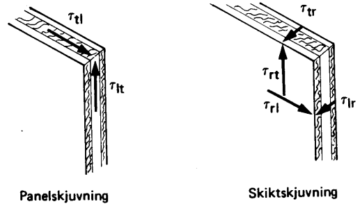
Figur 27:213 a Skjuvpåverkan vid plywood: Panelskjuvning Skiktssjuvning
