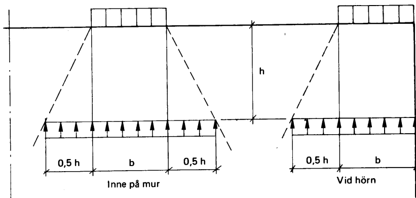
Figur 24:41 a Tryckutbredning under upplag.
