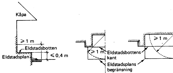
Figur 45:361 Eldstadsplan framför öppen spis. Vertikalsektion och plan
