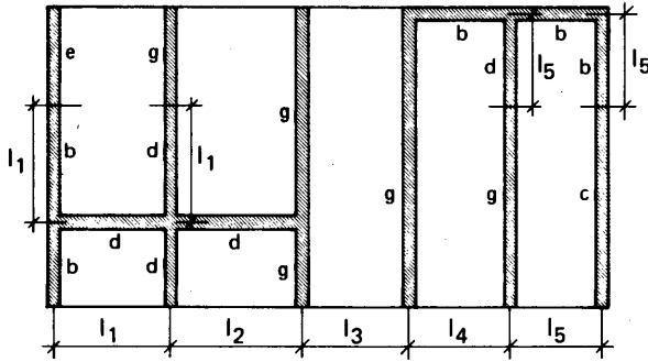
Figur 24:422 a Väggarpartier b, d, e och g för vilka nomogrammen i figurer 24:422 b – g gäller.
