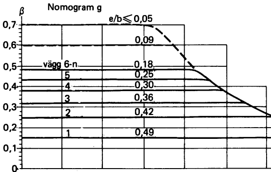
Figur 24:422 f–g Faktor vid väggar med från båda sidor anslutande bjälklag (innerväggar) eller då e/b är känt.
