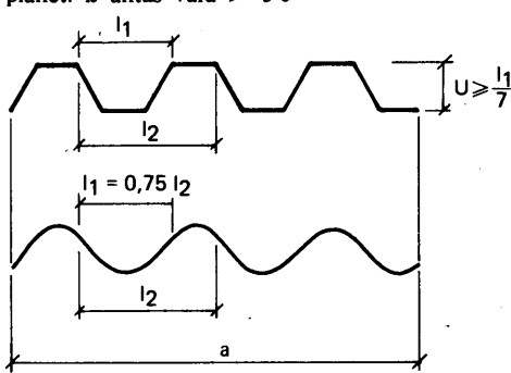
Figur 21:635 a Yta med tvärställda ribbor eller korrugeringar. Beteckningar för beräkning av tangentiell vindlast.
