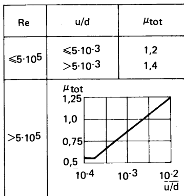
Figur 21:6341 b Formfaktorer för cylindriska stänger med l > 5 d . Re är Reynolds tal och u är ojämnheters höjd över omgivande yta.
