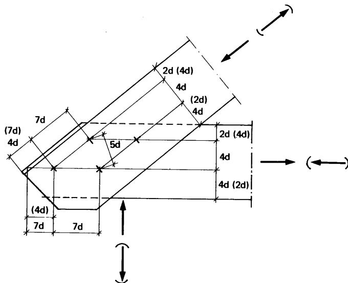
Figur 27:224 Minimiavstånd mellan skruvar och från skruv till virkeskant i skruvförband utan mellanläggsbrickor. Värderna inom parentes gäller för inom parentes angiven kraftpåverkan.
