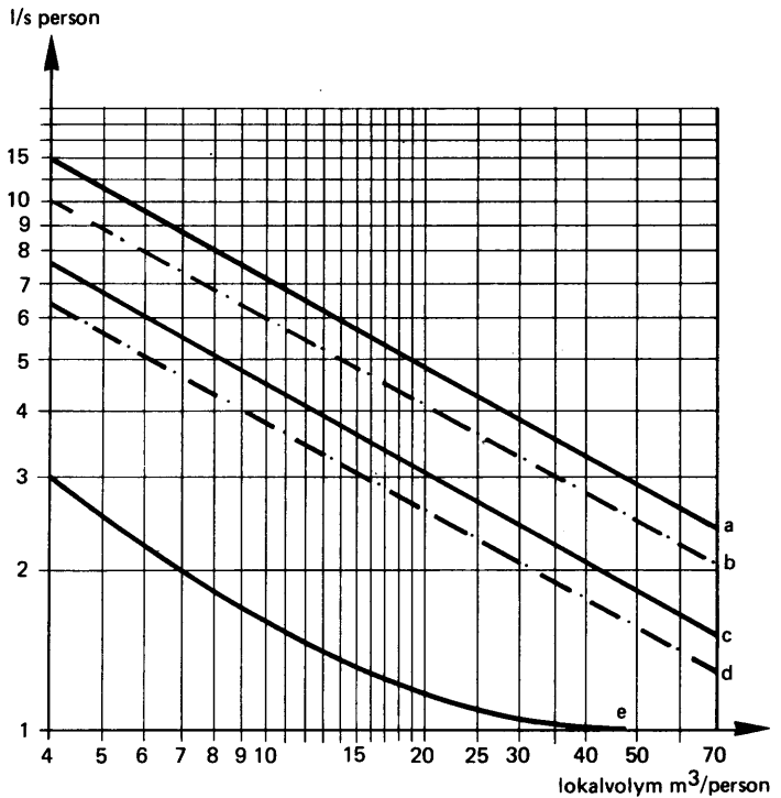
Figur 36:22 Godtagna uteluftsflöden.
