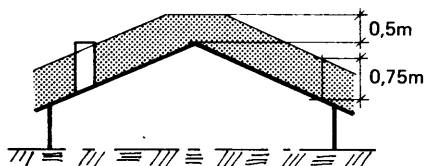
Figur 36:43 Ventilationsskorstens höjd över tak vid självdragsventilation.
