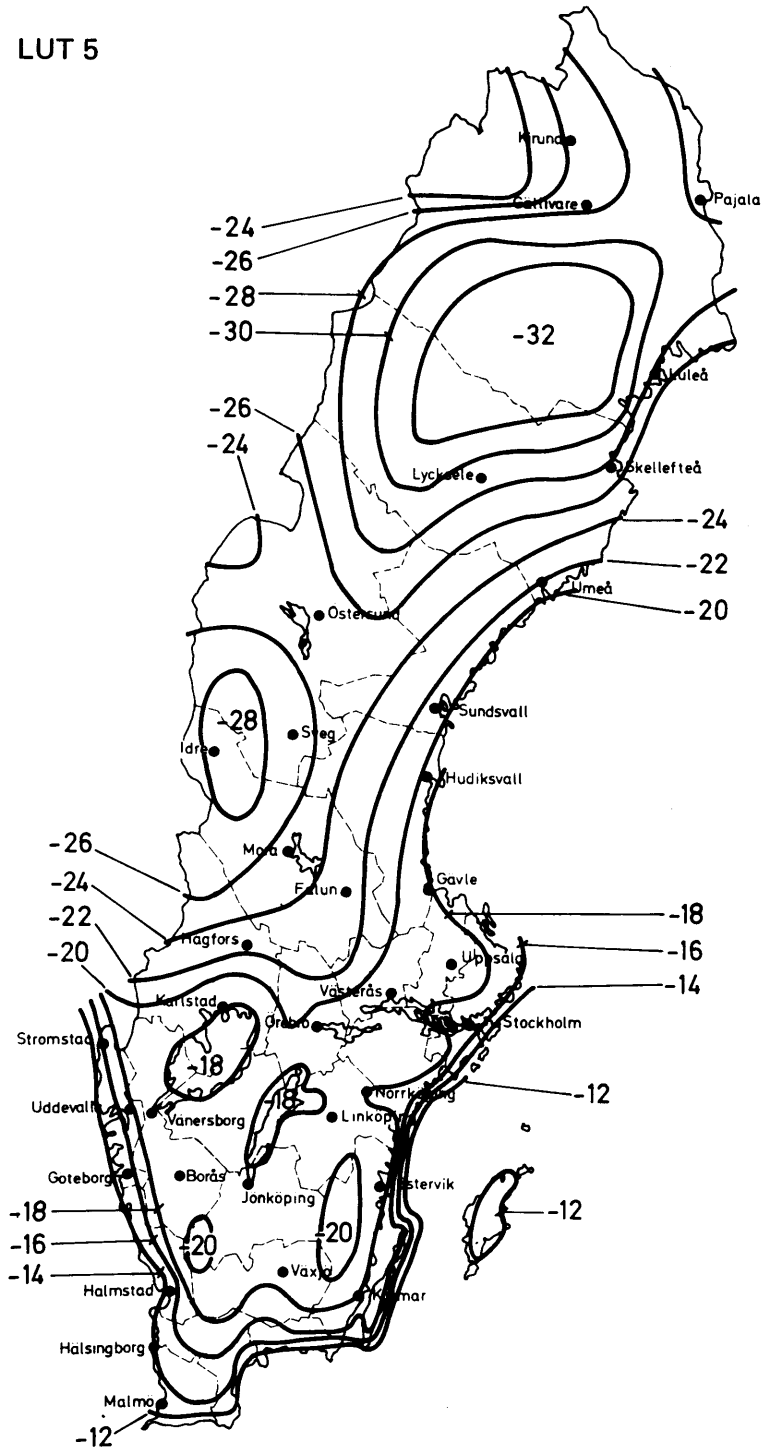
Figur 35:23 b Isotermkarta visande dimensionerande lägst utetemperatur för hus av sten eller annan tung byggnad, LUT 5. LUT-värden enligt figuren korrigeras om ifrågasatt byggnad ligger på en plats som bedöms vara kallare eller varmare än trakten i genomsnitt.
