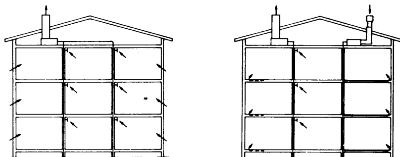
Typ F Ventilation med fläktstyrda frånluftsflöden
