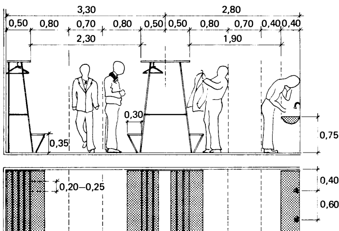
Figur 64:3 b Minsta godtagbara fria utrymmen vid klädställning och tvättränna. Mått i meter.
