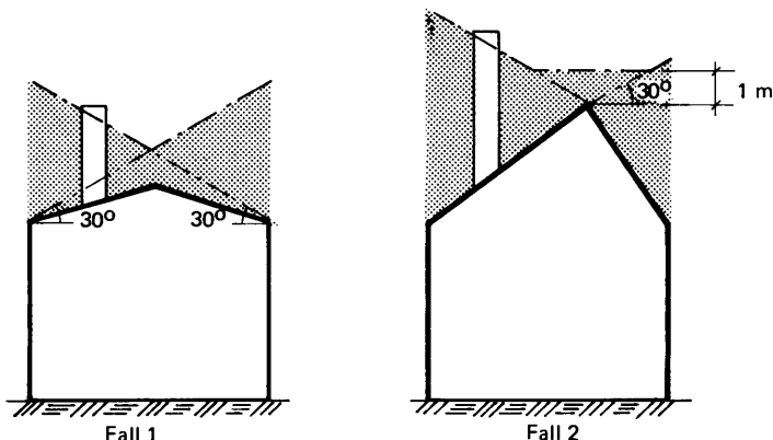
Figur 44:1222 Beräkning av höjd för rökkanal till panncentral med tillförd värmeeffekt 0,06 < P \leq 50 MW, tunnlolja.
