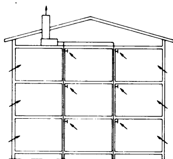
Typ F Ventilation med fläktstyrda frånluftsflöden
