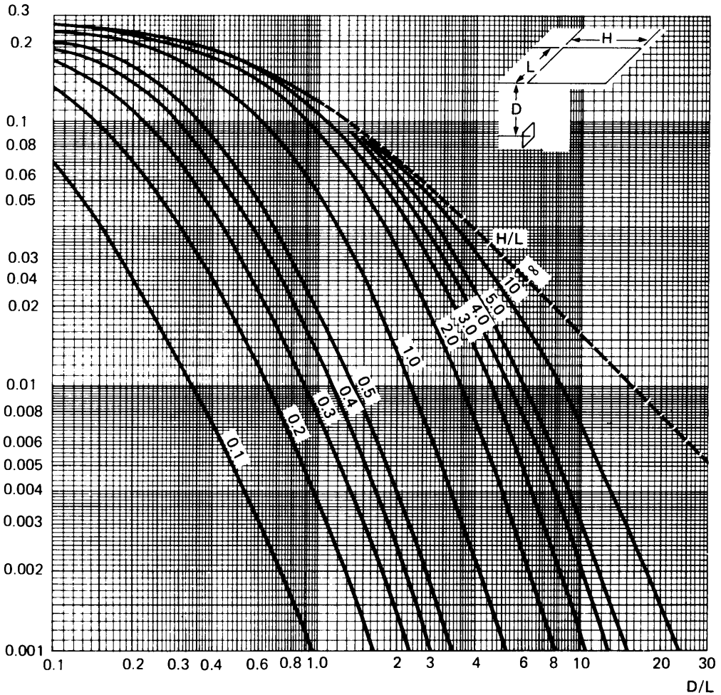
Figur 35:22 c Vinkelkoefficienten \varphi vid strålning mellan en liten yta och en mot denna vinkelrät större yta.
