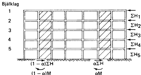
Figur 22:44 b Plan och längdsnitt genom en byggnadsstomme för flervåningsbyggnad. Figuren visar i byggnadens längdled verkande horisontalkrafter H. Varje pil betecknar en H-kraft där ej annat anges. Lutande streckmarkering betecknar i horisontalled stabiliserande konstruktion. \Sigma H_v betecknar summan av H-kraften under bjälklag v.
