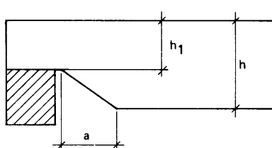
Figur 27:332 Inskäring vid upplag.
