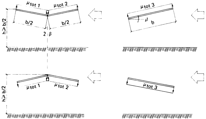
Figur 21:6344 Formfaktor \mu_{tot} för skärmtak som lutar vinkeln \beta mot horisontalplanet. \beta antas vara > 5^\circ .
