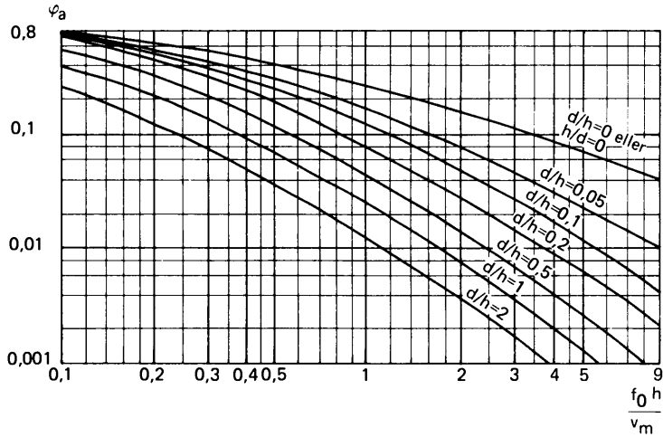
Figur 21:642 d Vindlastens storleksfaktor som funktion av f_0 h/v_m med egenfrekvensen för grundsvängningen f_0 , den anblåsta konstruktionens höjd h , dess största tvärrmått d och vindens medelhastighet v_m .
