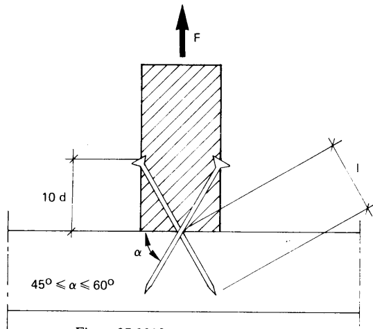
Figur 27:2223 b Skråspikning.
