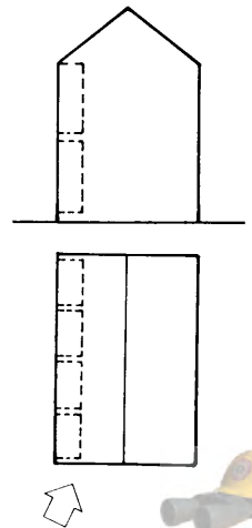
Figur 21:6344 Formfaktor \mu_{tot} för skärmtak som lutar vinkeln \beta mot horisontalplanet. \beta antas vara > 5^\circ .
