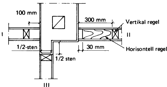
Figur 44:324 a Väggsanslutningar till rökkanals omslutningsvägg. Vid alternativ I (vägg med vertikala regler) skall regel befinna sig minst 100 mm från rökkanalens omslutningsvägg. Vid alternativ II (vägg med horisontella regler) skall ändtytor på regler befinna sig minst 30 mm från omslutningsväggen och eventuell vertikal regel e d minst 300 mm från väggen. Vid alternativ III får såväl väggpanel som träregel anslutas direkt mot murklock.
