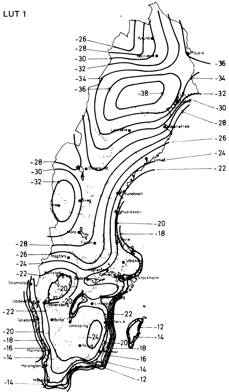
Figur 35:23 a Isotermkarta visande dimensionerande lägsta utetemperatur för hus av trä eller annan lätt byggnad, LUT 1. LUT-värden enligt figuren korrigeras om ifrågasvarande byggnad ligger på en plats som bedöms vara kallare eller varmare än trakten i genomsnitt.
