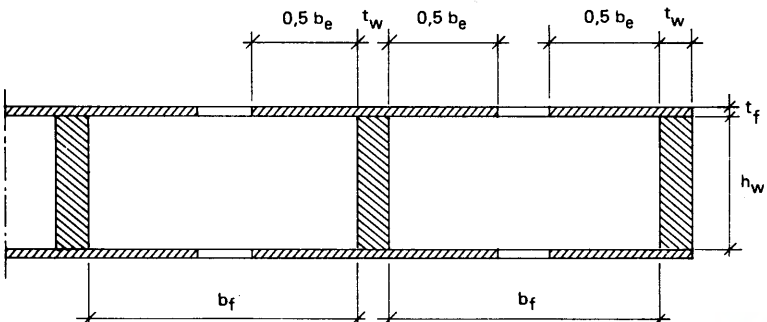
Figur 27:334 Balk med flänsar av skivmaterial.
