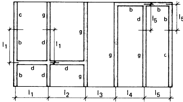
Figur 24:422 a Väggarpartier b, c, d och g för vilka nomogrammen i figurer 24:422 b - g gäller.
