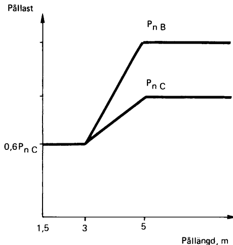
Figur 23:6526 Tillåten pållast för olika pållängd. P_{nB} normerad last för betongpåle i klass B. P_{nC} normerad last för betongpåle i klass C eller last för stålpåle med tvärsnittsytan > 0,01 m 2 eller för träpåle enligt :652.
