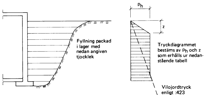
Figur 21:451 Jordtryck vid packad återfyllning av friktionsjord.
