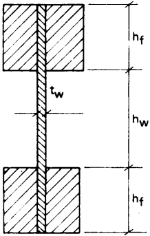
Figur 27:334 Balk med flänsar av konstruktionsvirke och liv av skivmaterial.
