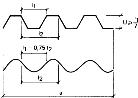
Figur 21:635 a Yta med tvärställda ribbor eller korrugeringar. Beteckningar för beräkning av tangentiell vindlast.
