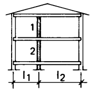
Figur 24:422 d - e Faktor vid väggar med från båda sidor anslutande bjälklag (innerväggar).
