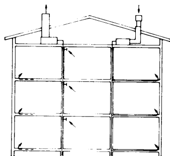
Typ FT Ventilation med fläktstyrda till- och frånluftsflöden
