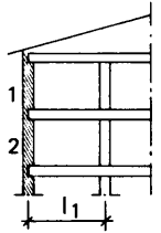
Figur 24:422 b - c Faktor vid väggar med från en sida anslutande bjälklag (ytterväggar och liknande). Nomogram b gäller vid korsarmade bjälklag med minsta spännvidden max 5,0 m. Nomogram c gäller vid enkelspända bjälklag \leq 5,0 m.
