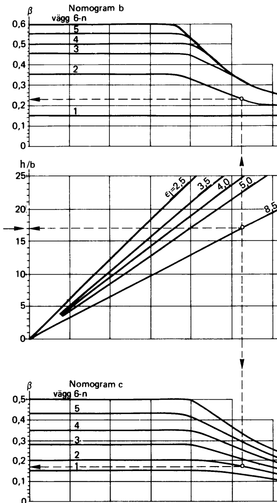
Figur 24:422 b - c Faktor vid väggar med från en sida anslutande bjälklag (ytterväggar och liknande). Nomogram b gäller vid korsarmade bjälklag med minsta spännvidden max 5,0 m. Nomogram c gäller vid enkelspända bjälklag \leq 5,0 m.
