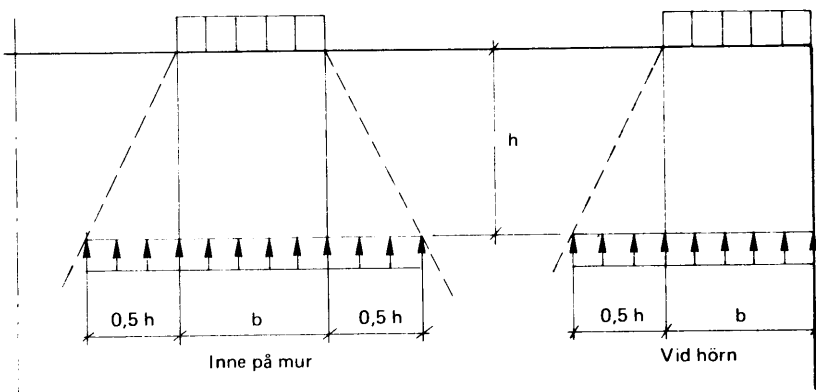
Figur 24:41 a Tryckutbredning under upplag.
