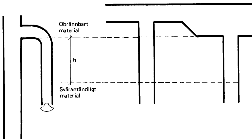
Figur 52:342 b Princip för anordnande av röklås.
