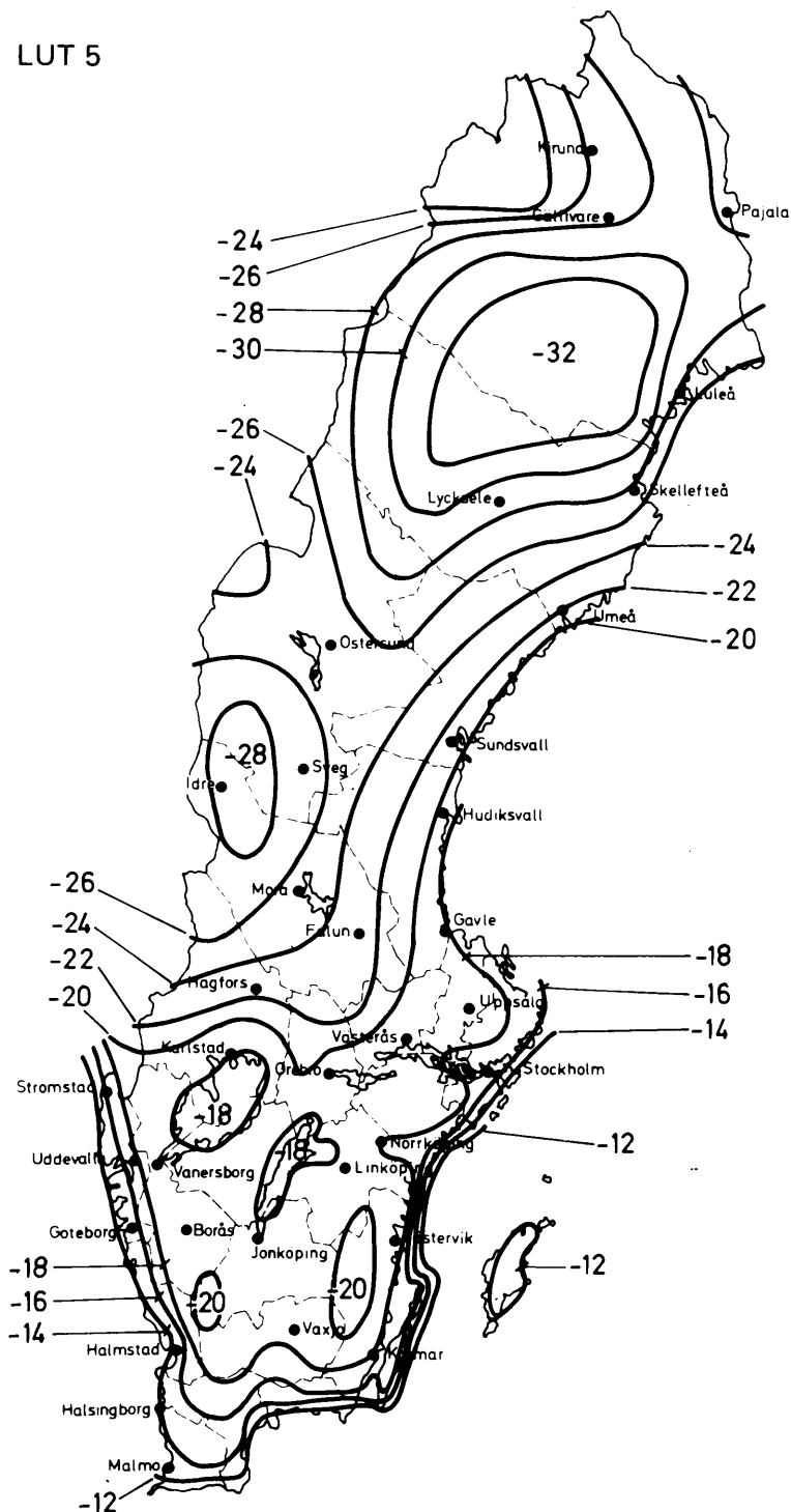
Figur 35:23 b Isotermkarta visande dimensionerande lägst utetemperatur för hus av sten eller annan tung byggnad, LUT 5. LUT-värden enligt figuren korrigeras om ifrågasvarande byggnad ligger på en plats som bedöms vara kallare eller varmare än trakten i genomsnitt.
