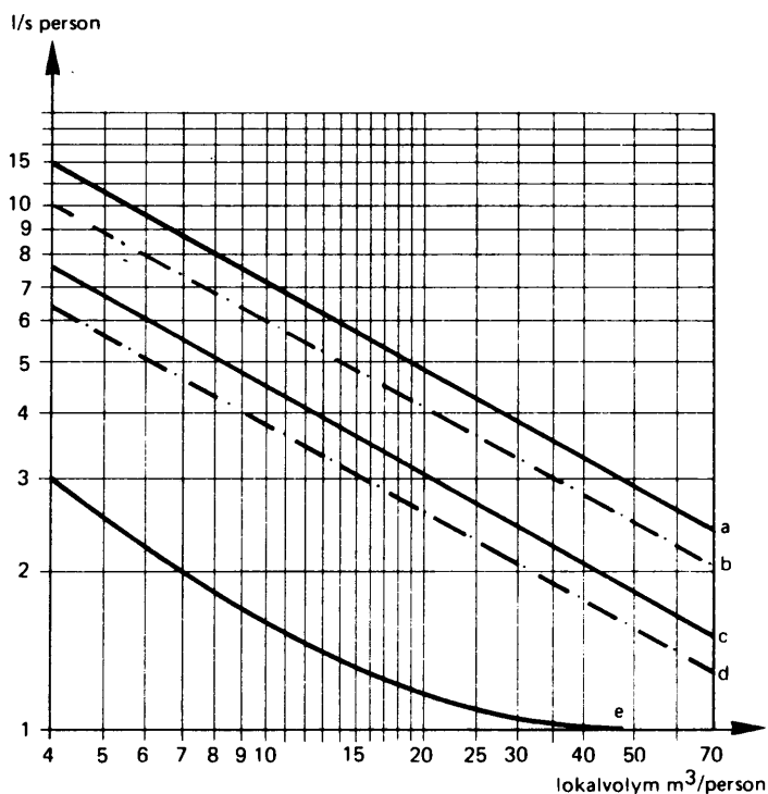
Figur 36:22 Godtagna uteluftsflöden.
