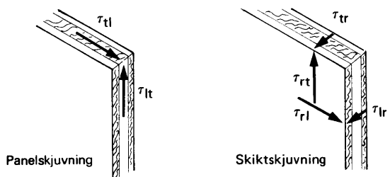
Figur 27:213 a Skjuvpåverkan vid plywood: Panelskjuvning Skiktskjuvning
