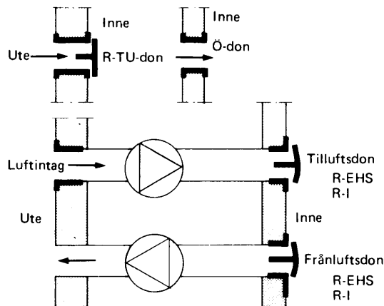
Figur 36:42 Förklaring av benämningar på don.
