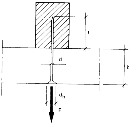
Figur 27:2223 a Dragen spik.
