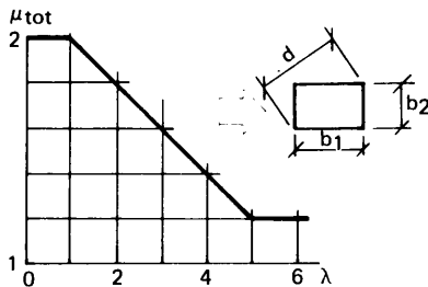
Figur 21:6341 a Formfaktorer för rektangulära stänger med l > 5d och \lambda = b_1/b_2 .
