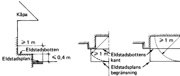
Figur 45:361 Eldstadsplan framför öppen spis. Vertikalsektion och plan
