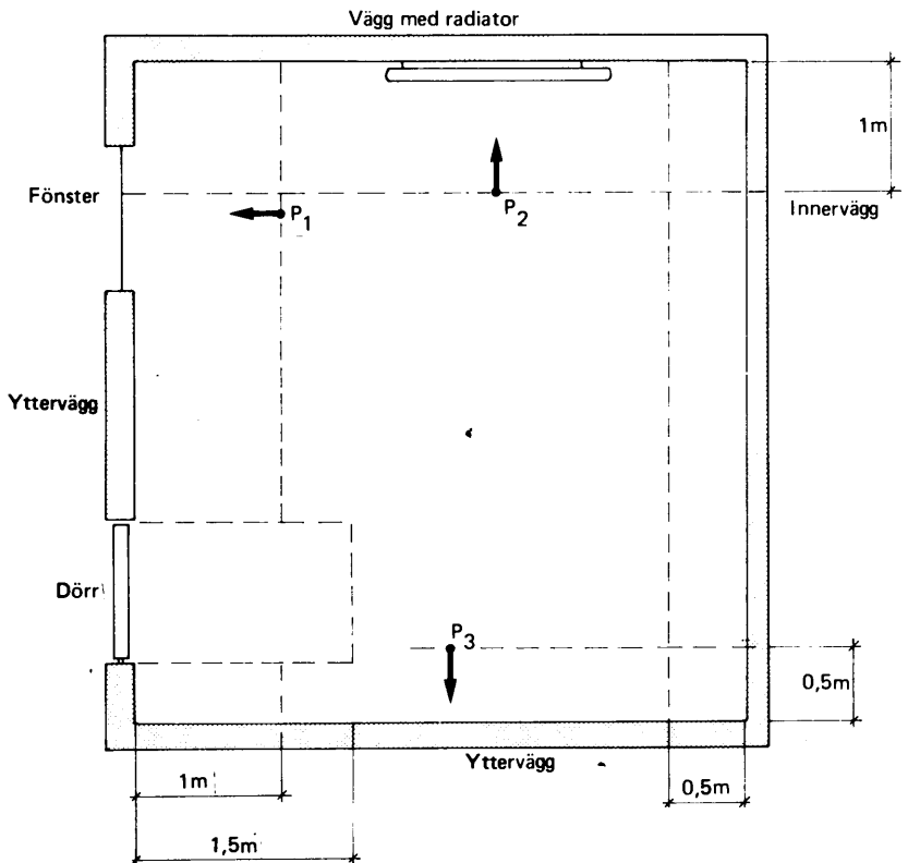
Figur 35:21 Exempel som visar kontrollzonens storlek och placering av punkter P_1 – P_3 enligt :231.
