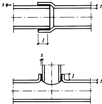
Rak överlappsfog.
