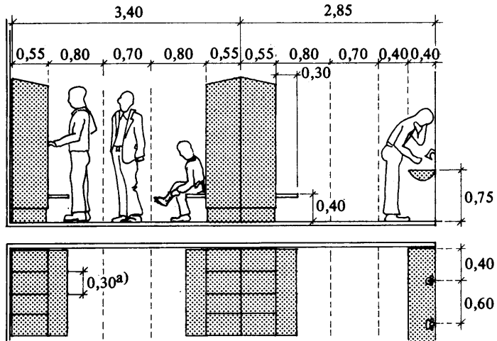
Figur 64:3 b. Exempel på minsta godtagna fria utrymmen vid klädskåp med sittbänk och tvättränna. – a) Vid åtskillnad mellan gång- och arbetskläder fordras större sammanlagd skåpbredd.
