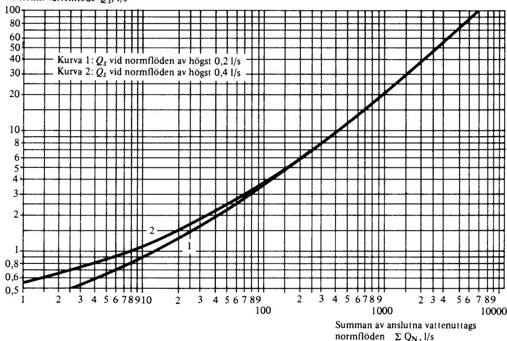
Figur 51:151. Godtaget sannolikt vattenflöde för fördelningsledning i bostäder, kontor o d. Speciellt vid mindre värden på sannolikt flöde bör detta kontrolleras, så att det inte blir mindre än det flöde som kan förväntas uppträda i ledningen.
