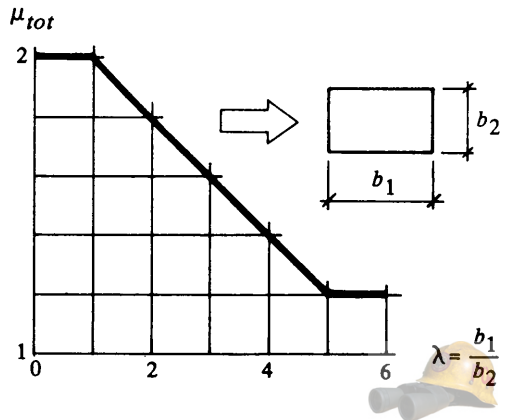
Figur 22:5341 a. Godtagna värden på formfaktorn \mu_{tot} för rektangulära stänger med l \geq 5 ggr diagonalmättet.
