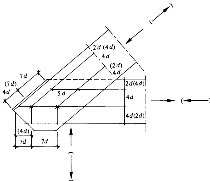
Figur 27:54. Förutsatta minimialavstånd mellan skruvar och från skruv till virkeskant i skruvförband utan mellanläggsbrickor. Värderna inom parentes gäller för inom parentes angiven kraftpåverkan. ( d är skruvdiameter.)
