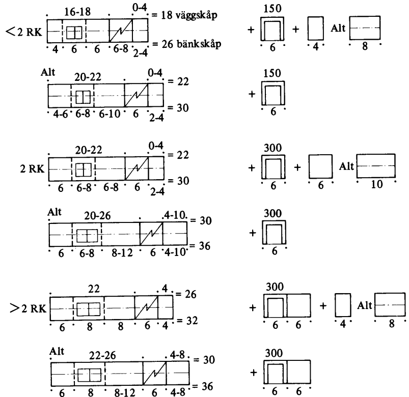
Figur 71:214. Delmått på godtagen minsta inrednings- och utrustningsmängd för olika lägenhetsstorlekar. Delmått anges i dm. 150 och 300 anger kyld volym i liter.
