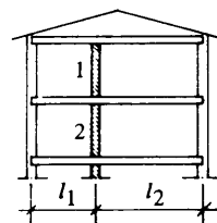
Figur 24:422 d-e. Godtagna reduktionsfaktorer för väggar med från båda sidor anslutande bjälklag (innerväggar).
