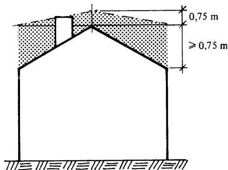
Figur 44:121 a. Godtagen höjd över yttertak för rökkanal, om ansluten eldstad har en tillförd värmeeffekt av högst 60 kW.
