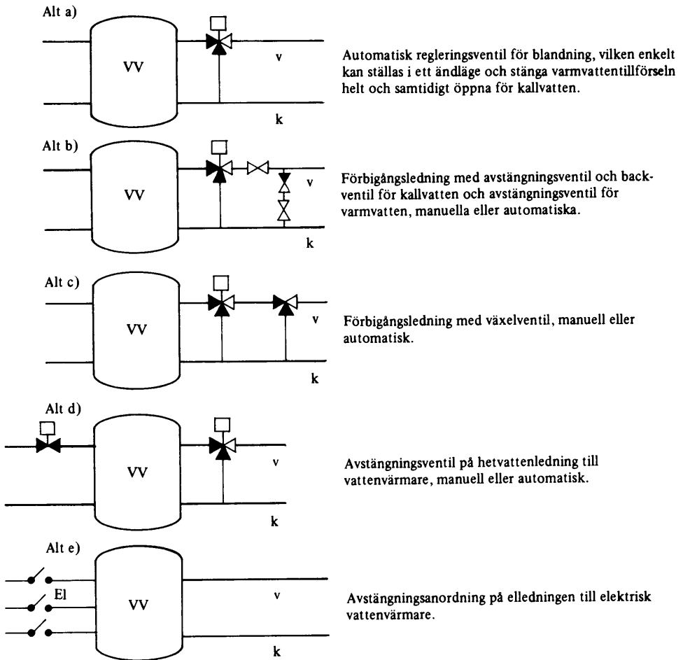
Figur 51:1662. Exempel på godtagget anordnande av kriskoppling.
