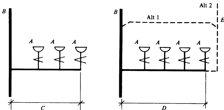
Figur 51:261 b. Exempel på luftning av ledning
