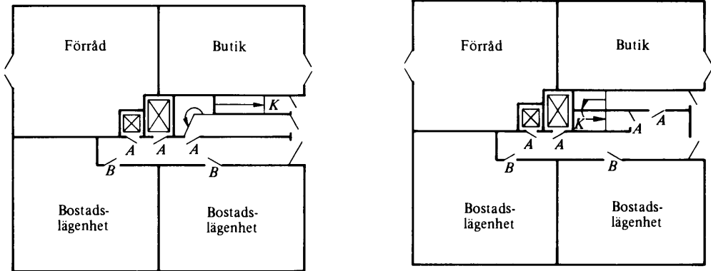
Figur 37:126. Principsskisser med exempel på entréväning vid brandsäkert trapphus i bostadshus. A betecknar dörr i lägst klass A60, B dörr i lägst klass B30 och K betecknar källartrappa.
