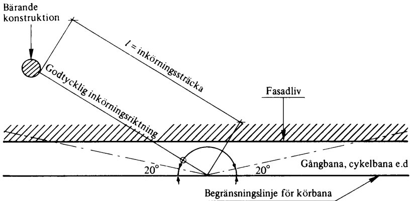
Figur 22:82 b. Antagna inkörningsriktningar och inkörningssträckor.
