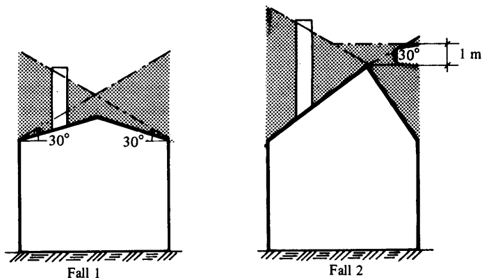
Figur 44:1222. Godtagen beräkning av höjd för rökkanal till anläggning avsedd för tunnolja, med tillförd värmeeffekt 0,06 < P \leq 50 MW. Principskiss. Av figurens nivålinjer framgår lägsta godtagbara höjd.
