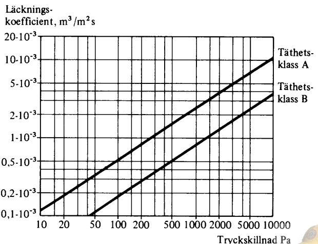
Figur 52:21a. Godtagna täthetsklasser för inomhus förlagda kanaler.
