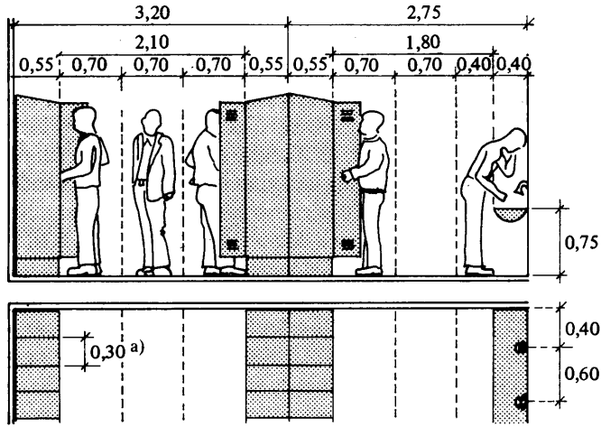
Figur 64:3 a. Exempel på minsta godtagna fria utrymmen vid klädskåp och tvättränna. – a) Vid åtskillnad mellan gång- och arbetskläder fordras större sammanlagd skåpbredd.
