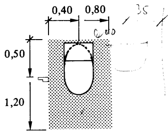
Figur 63:21 c. Wc-stol eller bidé (0,40 × 0,70 m).
