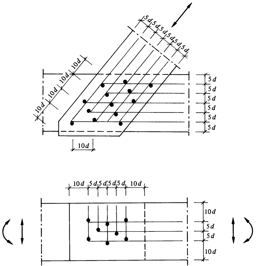
Figur 27:52 a. Förutsatt minimiavstånd mellan spikar och från spik till kant för virke och K-skivor och till virkesände ( d är spikens tvärmått). Där två avstånd anges gäller det större.
