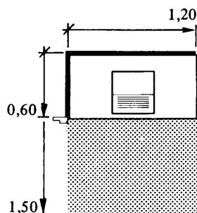
Figur 63:21 g. Tvättbänk (1,00 × 0,60 m och 1,20 × 0,60 m).
