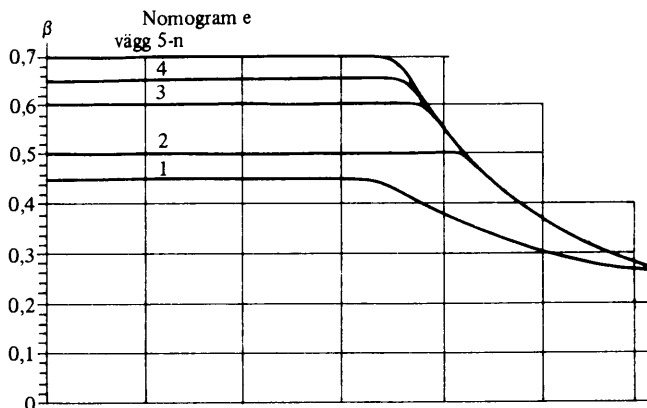
Figur 24:422 d-e. Godtagna reduktionsfaktorer för väggar med från båda sidor anslutande bjälklag (innerväggar).
