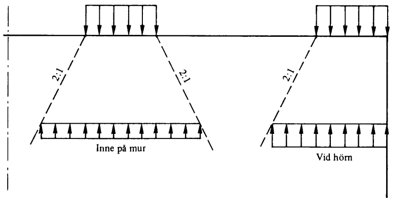
Figur 24:41 a. Godtagen tryckutbredning under ett upplag.
