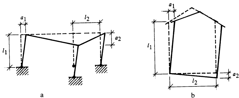
Figur 21:313 a och b. Exempel på lutningsändringar hos systemlinjer för bygnadsdelar. Lutningsändringen a_1/l_1 gäller för vertikala bärvverk och a_2/l_2 för horisontella.
