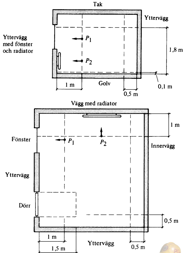
Figur 35:21. Exempel som visar kontrollzonens storlek och placering av punkterna P_1 och P_2 enligt :21.
