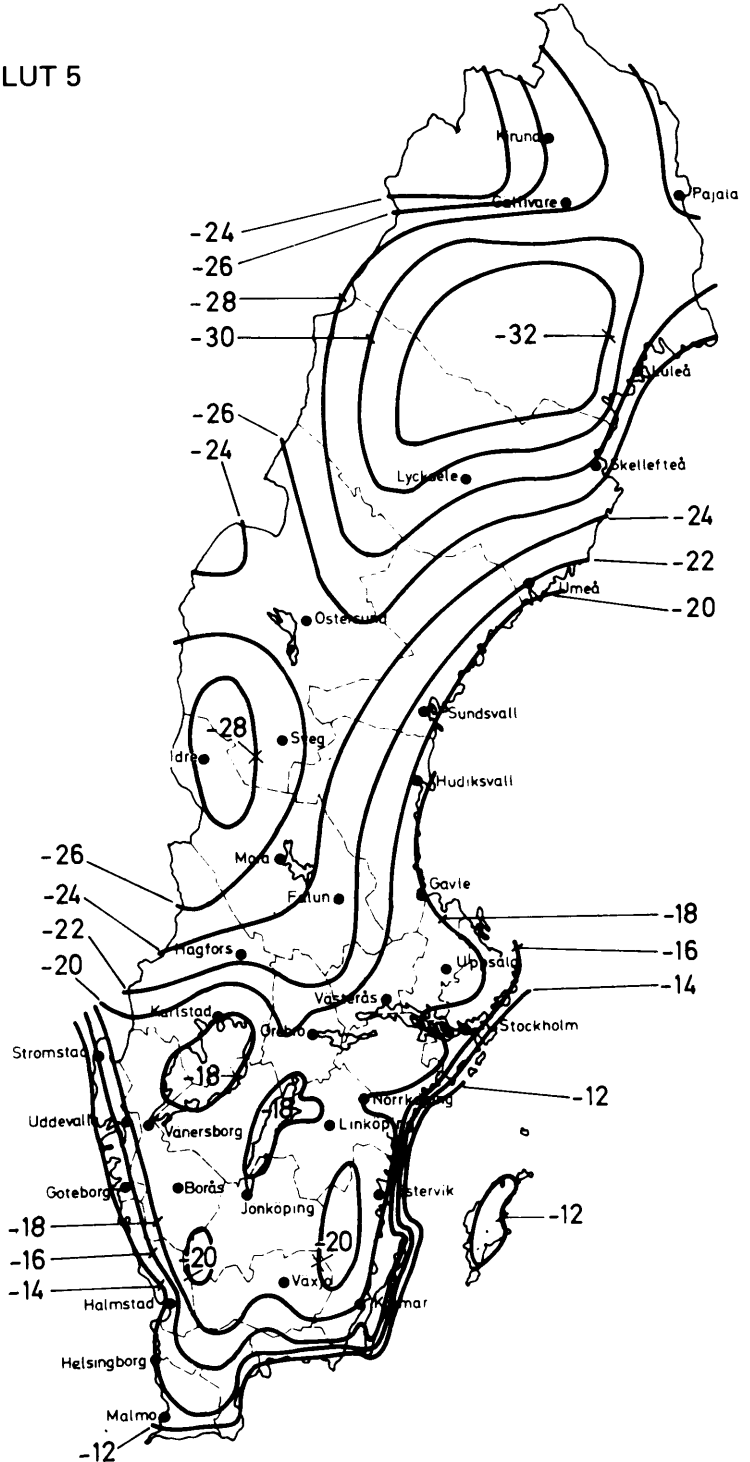
Figur 35:23 b. Isotermkarta som visar den dimensionerande lägsta utetemperaturer för hus av sten eller annan tung byggnad, LUT 5. LUT-värden enligt figuren korrigeras om ifrågasatt byggnad ligger på en plats som bedöms vara kallare eller varmare än trakten i genomsnitt.
