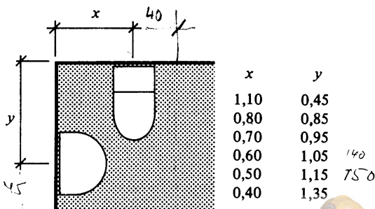
Figur 63:22. Exempel på godtagna kombinationsmått vid vinkeluppställning.
