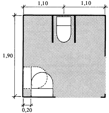
Figur 63:23 d. Tvättställ och wc-stol i utrymme för personer med låg rörlighet i rullstol, i utomhusrullstol eller som behöver hjälp vid toalettbesök. Tvättstället utflyttat 0,20 m från vägg. Streckad figur anger alternativt placering.
