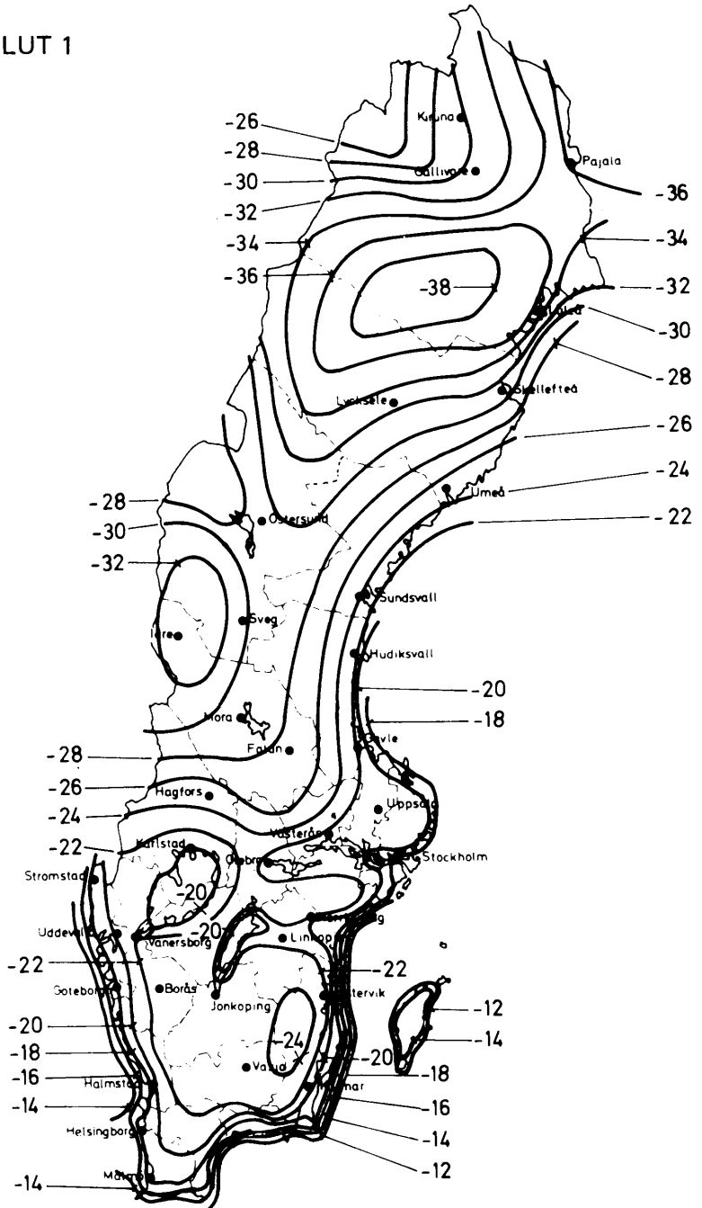
Figur 35:23 a. Isotermkarta som visar den dimensionerande lägsta utetemperaturer för hus av trä eller annan lätt byggnad, LUT 1. LUT-värden enligt figuren korrigeras om ifrågasvarande byggnad ligger på en plats som bedöms vara kallare eller varmare än trakten i genomsnitt.
