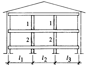
Figur 24:422 f-g. Godtagna reduktionsfaktorer för väggar med från båda sidor anslutande bjälklag (innerväggar) eller då e/b är känt. Nomogram f gäller vid enkelspända bjälklag i byggnader med två fack när l_1/l_2 \leq 0,8 och l_2 \leq 5,0 m. Nomogram g gäller vid enkelspända bjälklag i byggnader med tre eller flera fack med spannvidden högst 5 m samt där e bestäms enligt figuren.
