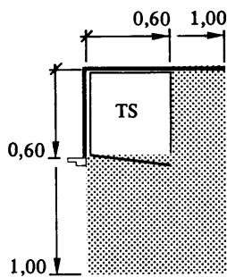
Figur 63:21 i. Torkskåp (0,60 × 0,60 m).
