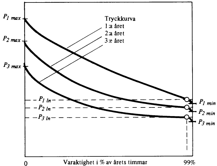
Figur 51:13. Definition av lägsta normala vattentryck.
