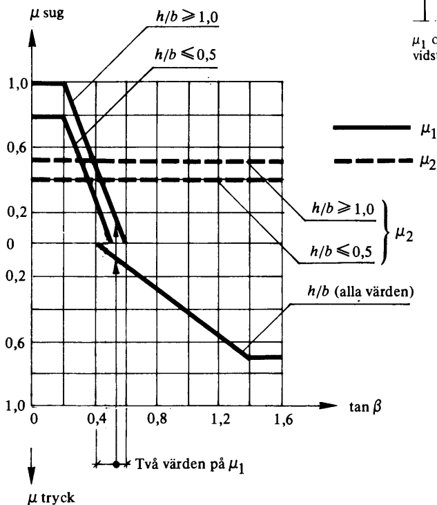
Figur 22:5332 a. Godtagna värden på formfaktorer för utvärdig vindlast på sadeltak. Om h/b är mellan 0,5 och 1,0 får värdet på \mu sug framtas genom interpolering. Vidare antas vindlasten vid viss taklutning ge såväl sug som tryck på den anblåsta sidan. A och B betecknar två olika lastfall, som båda förutsätts bli beaktade. Inverkan av motsatta vindriktningar förutsätts alltid bli prövade, se :51.
