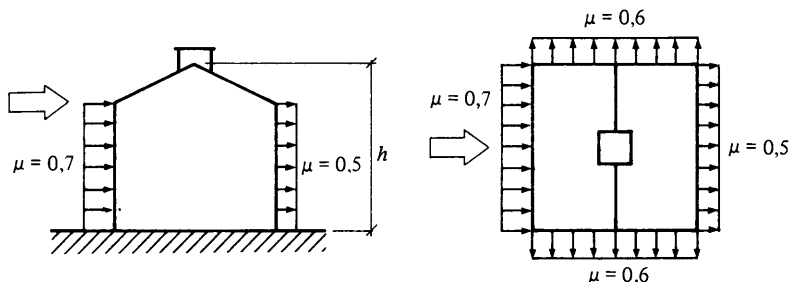
Figur 22:5331 a. Godtagna värden på formfaktorer för utvändigt vindlast på ytterväggar. Höjden h används för att bestämma det exceptionella hastighetstrycket enligt figur 22:52.
