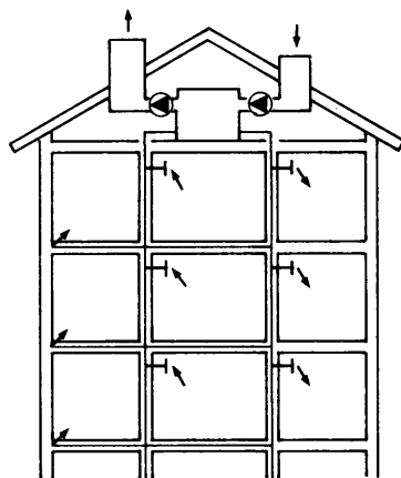
Typ FT Ventilation med fläktstyrda till- och frånluftsflöden
