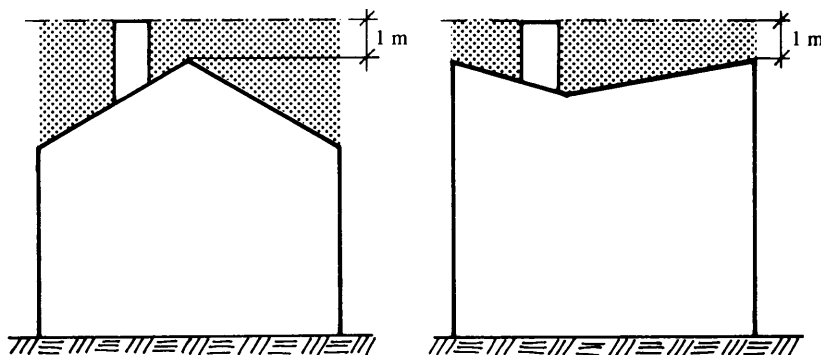
Figur 44:121 a. Godtagen höjd över yttertak för rökkanal, om ansluten eldstad har en tillförd värmeeffekt av högst 60 kW.
