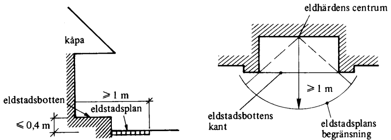
Figur 45:361. Eldstadsplan för öppen spis. Princip för minsta utsträckning. Vertikal-sektion och plan.
