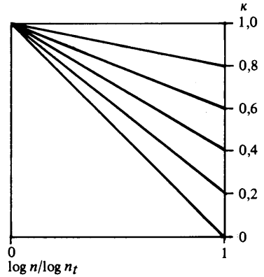
Figur 21:5213 b. Typiserade lastkollektiv.
