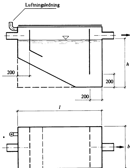
Figur 51:223 b. Godtagna dimensioner för oljeavskiljare och fettavskiljare (mm). Principskiss. Jfr tabell 51:223 d.
