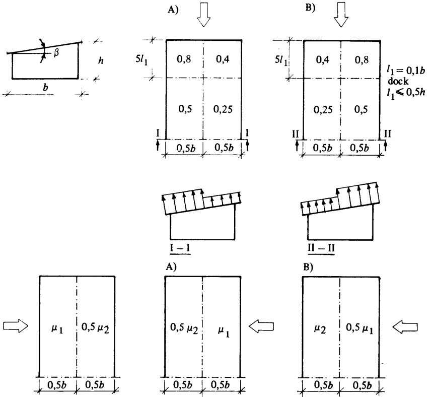
Figur 22:5332 b. Godtagna värden på formfaktorer för utvärdig vindlast på pulpettak. A och B betecknar två olika lastfall, vilka båda förutsatts bli beaktade. \mu_1 och \mu_2 bestäms enligt diagram i figur 22:5332 a.
