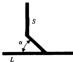
Stående SAMLINGSLEDNING (S) ansluten till liggande (L) med grenrör, \alpha \leq 45^\circ
