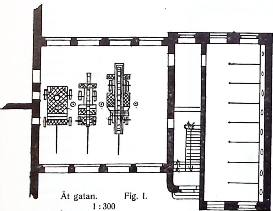
Spruthall och stall i en brandstation efter det gamla byggnadssättet i Berlin.
