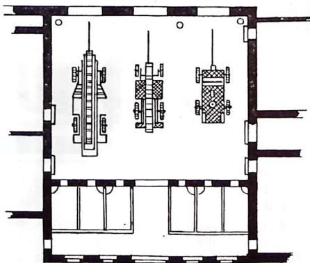
Spruthall i en brandstation efter amerikanskt byggnadssätt med utveckling på djupet.
