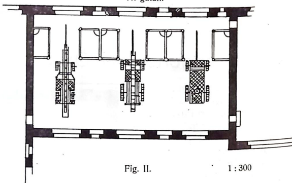
Spruthall i en brandstation efter amerikanskt byggnadssätt med utveckling på bredden.
