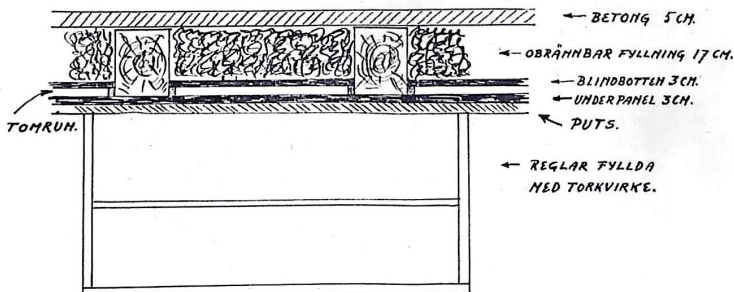
Bild 2. Schematisk genomskärning av mellanbotten.
