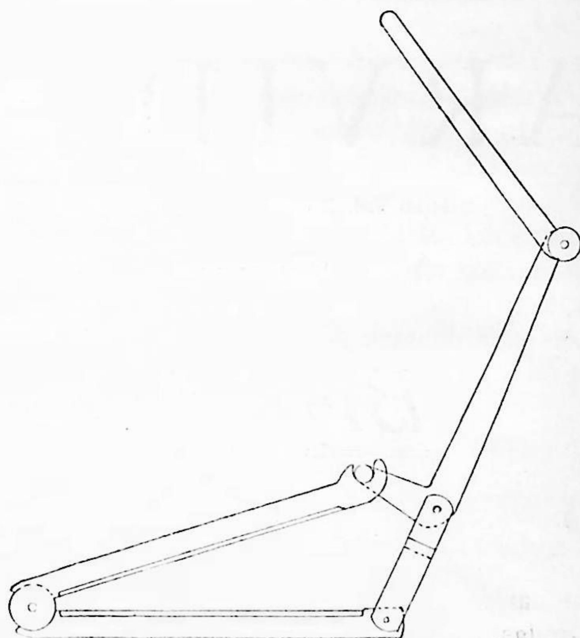
Slangklämman Enorm
