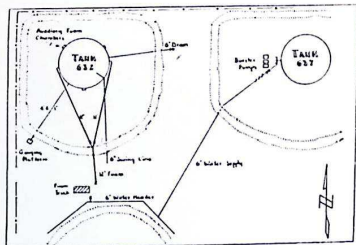
Bild 2. Subsurfaceförsökens arrangemang.
