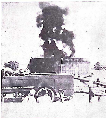
Bild 7. 3 min. efter släckningens början. Elden under kontroll.
