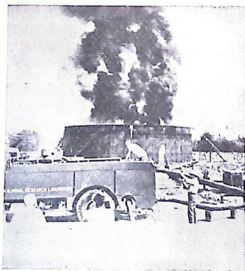
Bild 6. 1 min. 45 sek. efter släckningens början. Elden mattas.
