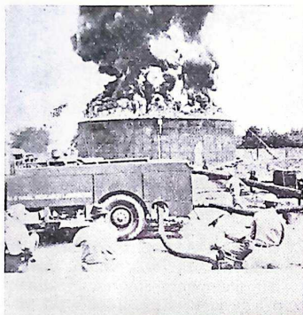
Bild 5. Branden 3 min. efter tändningen och omedelbart innan släckningen började.
